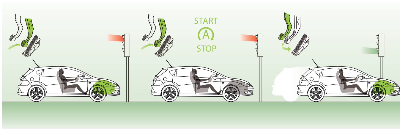
Funkce Start/Stop a systém rekuperace.
