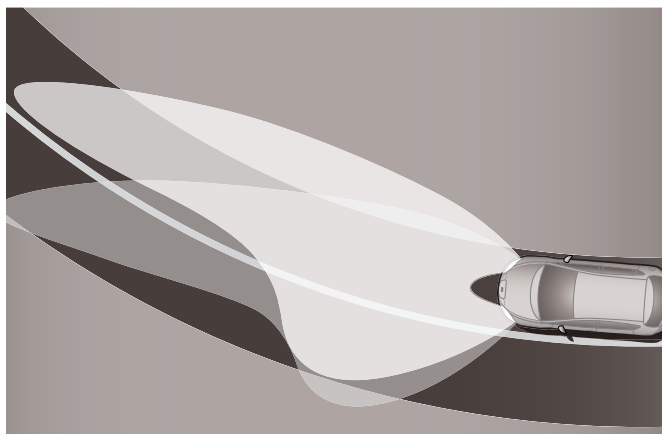
Natáčecí bi-xenonové světlomety.
